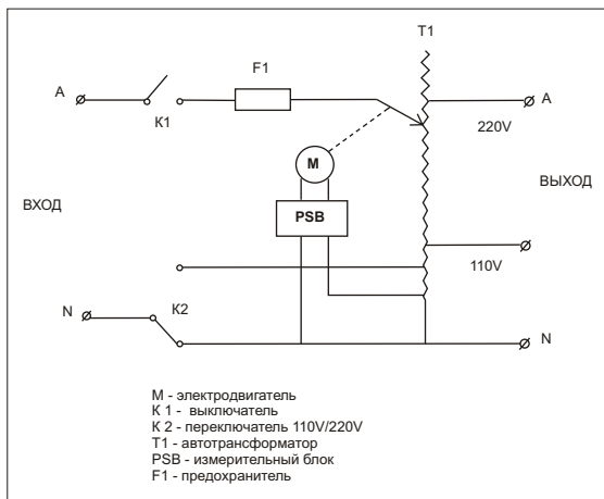
Схема устройства
